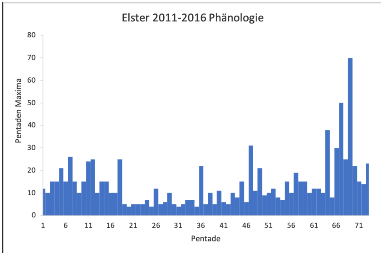
Abb. 2: Elster 2011-2016 Jahresverteilung
