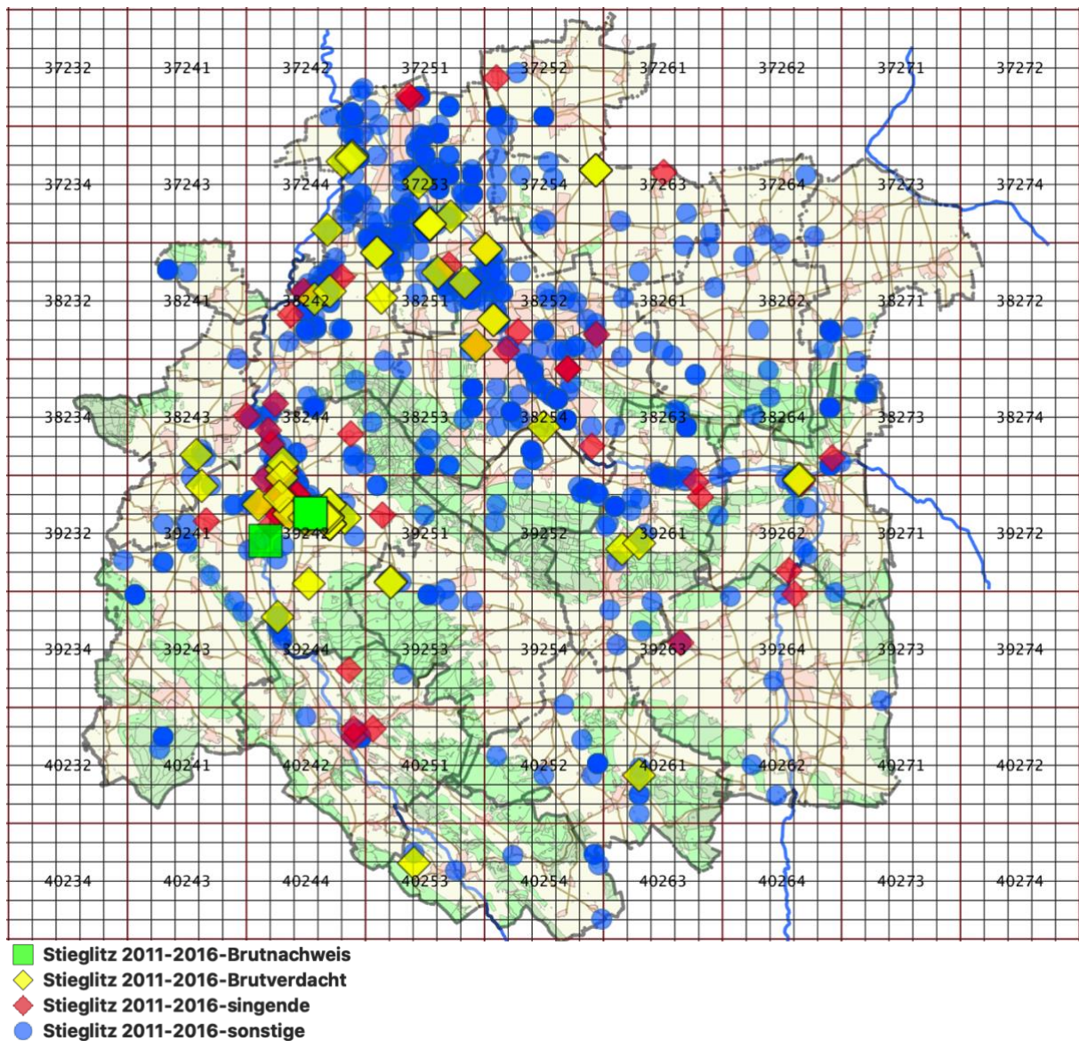
Abb. 1: Stieglitz 2011-2016 Verbreitung
